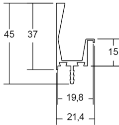
Doorsnede profiel
